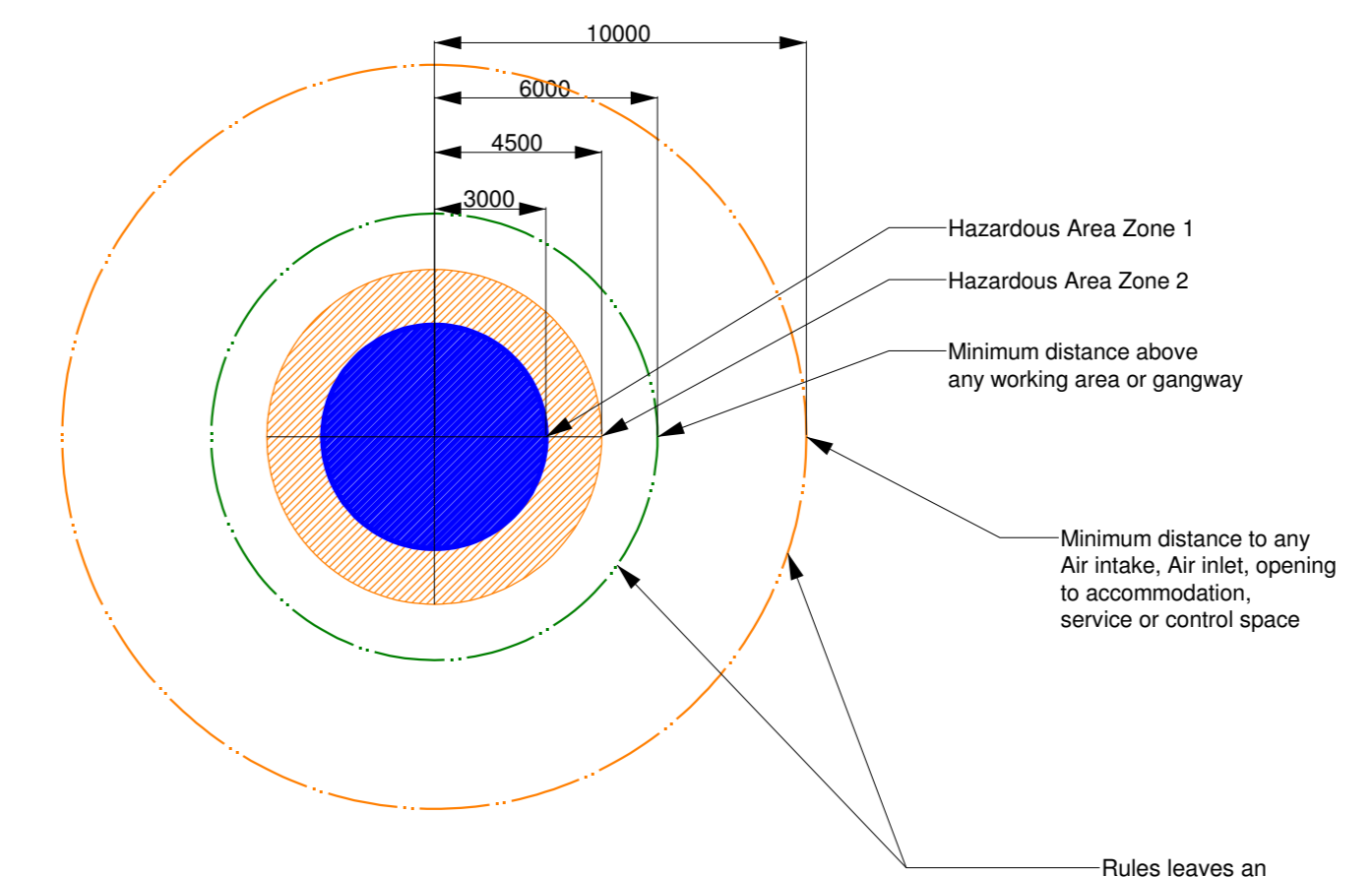
Vent mast
